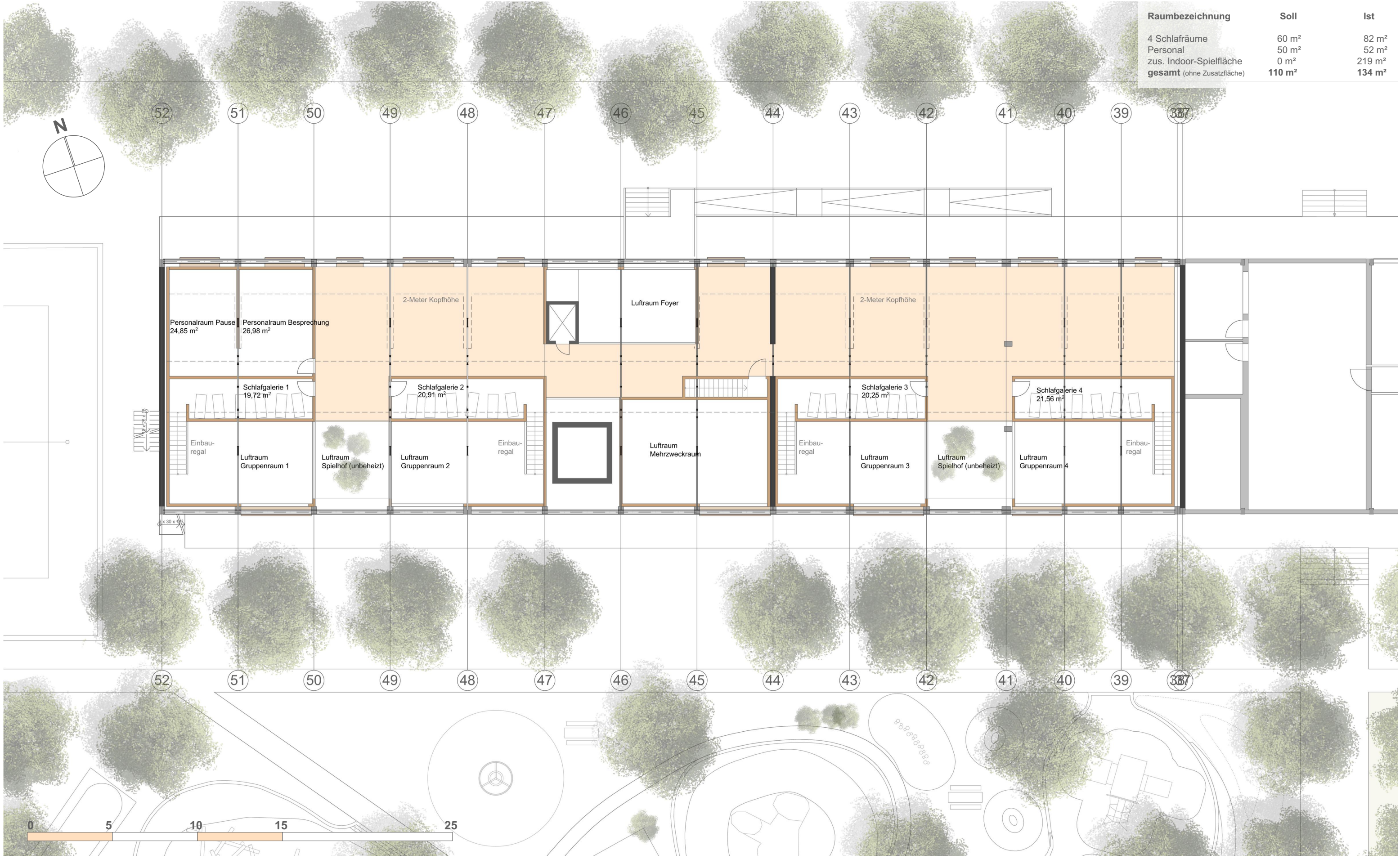
Grundriss OG 1:200
